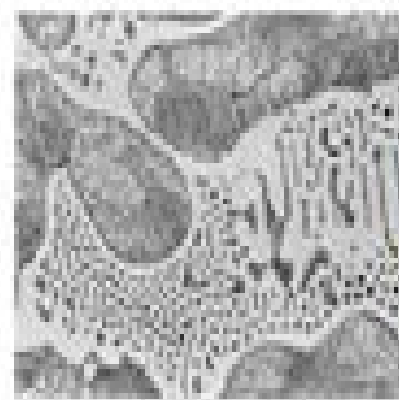
LEDEBURITA
