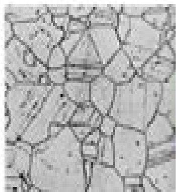
AUSTENITA
